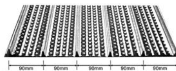
Hy-Rib (2 x 8)
